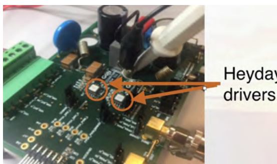
Carte d'évaluation de circuit imprimé avec 2 gate drivers Heyday alimentant des transistors en nitrure de gallium (GaN)
